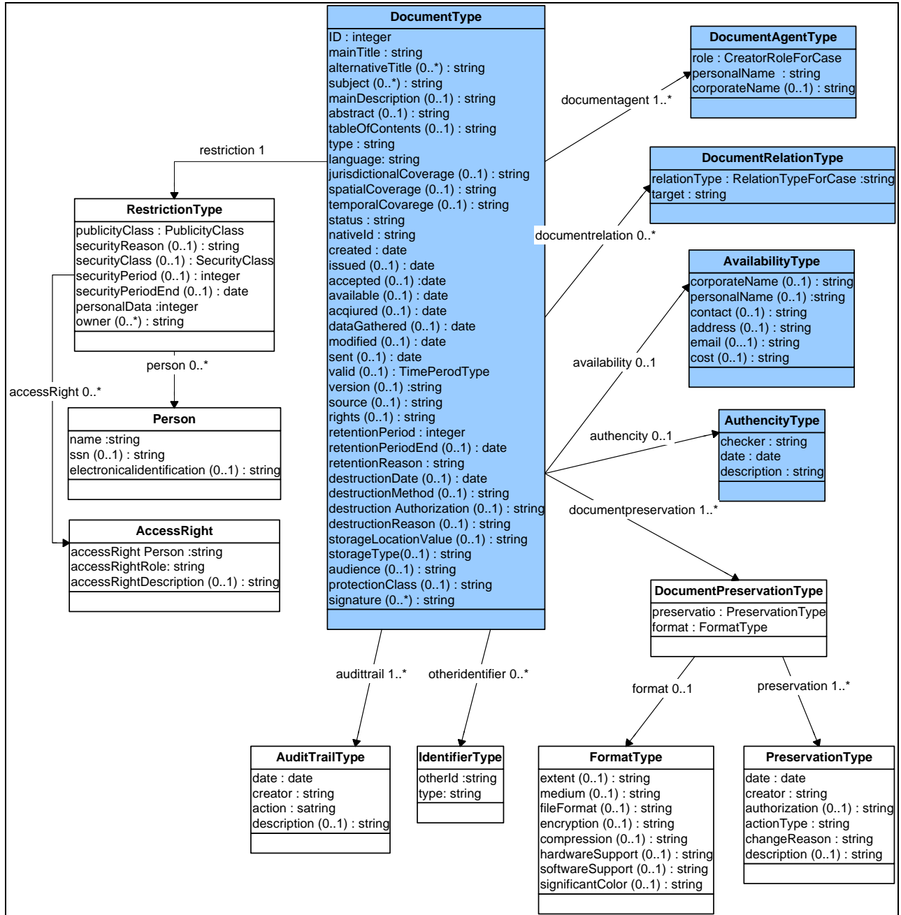
Kuva 3. Asiakirjan metatiedot UML-kaaviona
