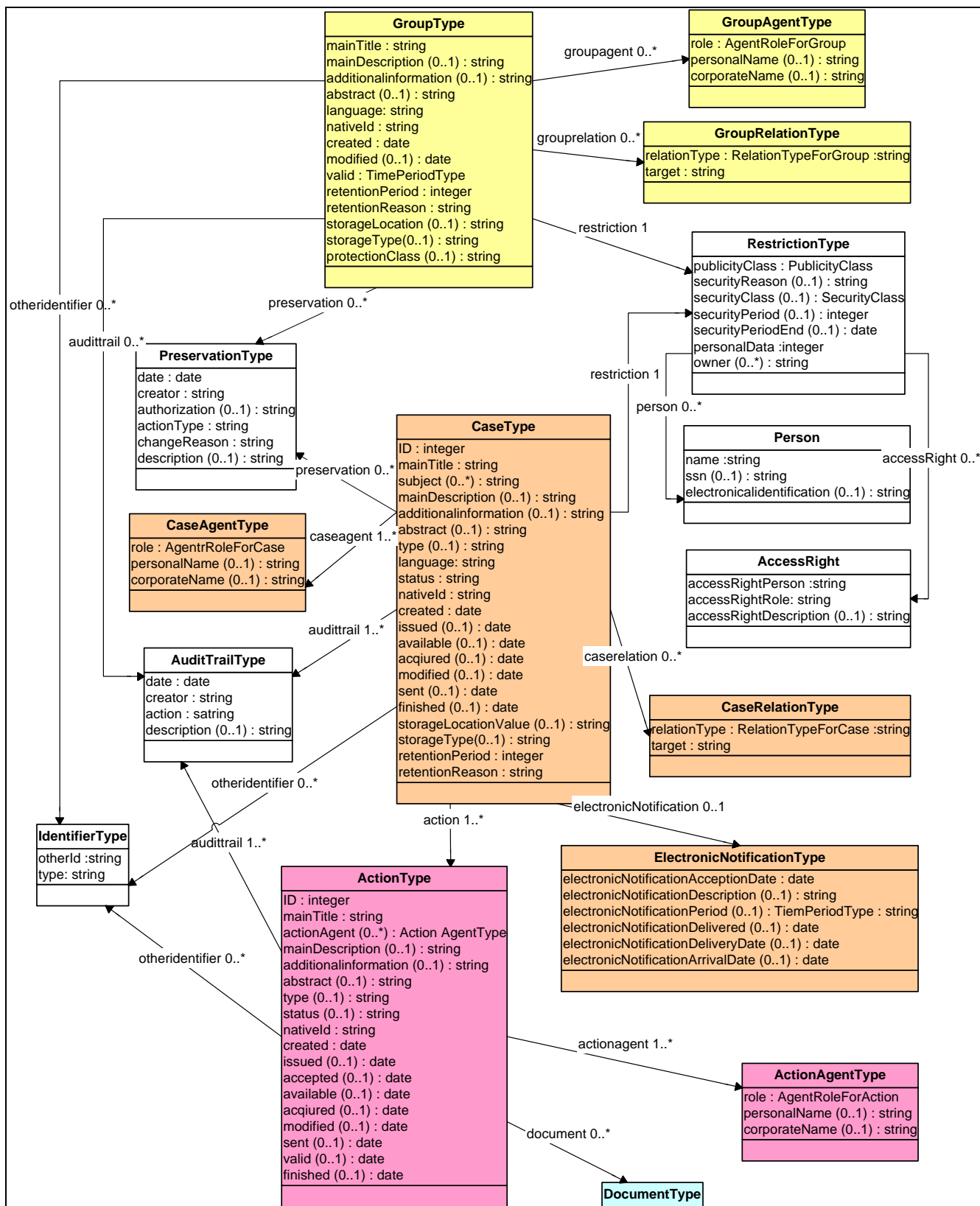
Kuva 2. Ryhmän, asian ja toimenpiteen metatiedot UML-kaaviona
