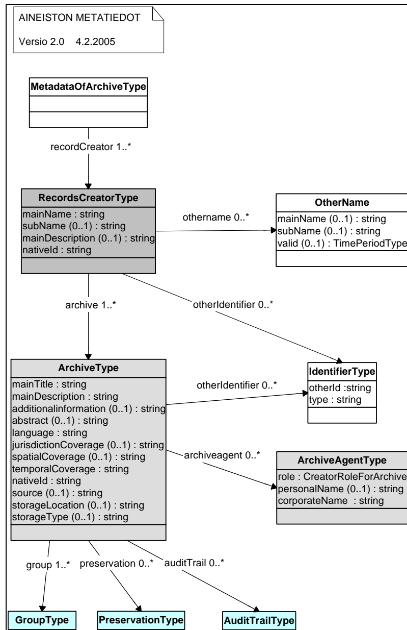
Kuva 1. Arkistonmuodostajan ja arkiston metatiedot UML-kaaviona
